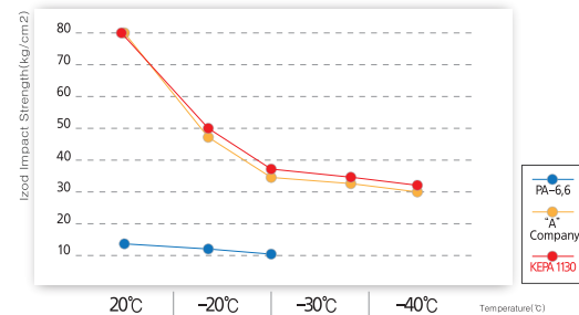
Nylon 6 / KEPA 1130 (80/20) Blendの低温衝撃強度Data
