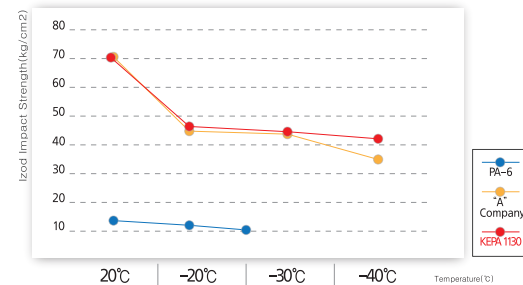
Nylon 6,6 / KEPA 1130 (80/20) Blendの低温衝撃強度Data
